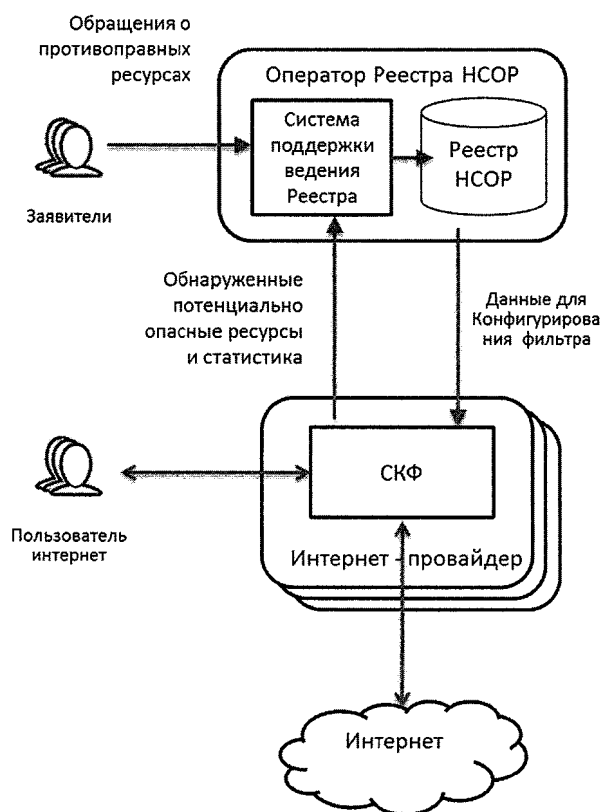
Рисунок 6. Принцип контроля доступа через Реестр НСОП
